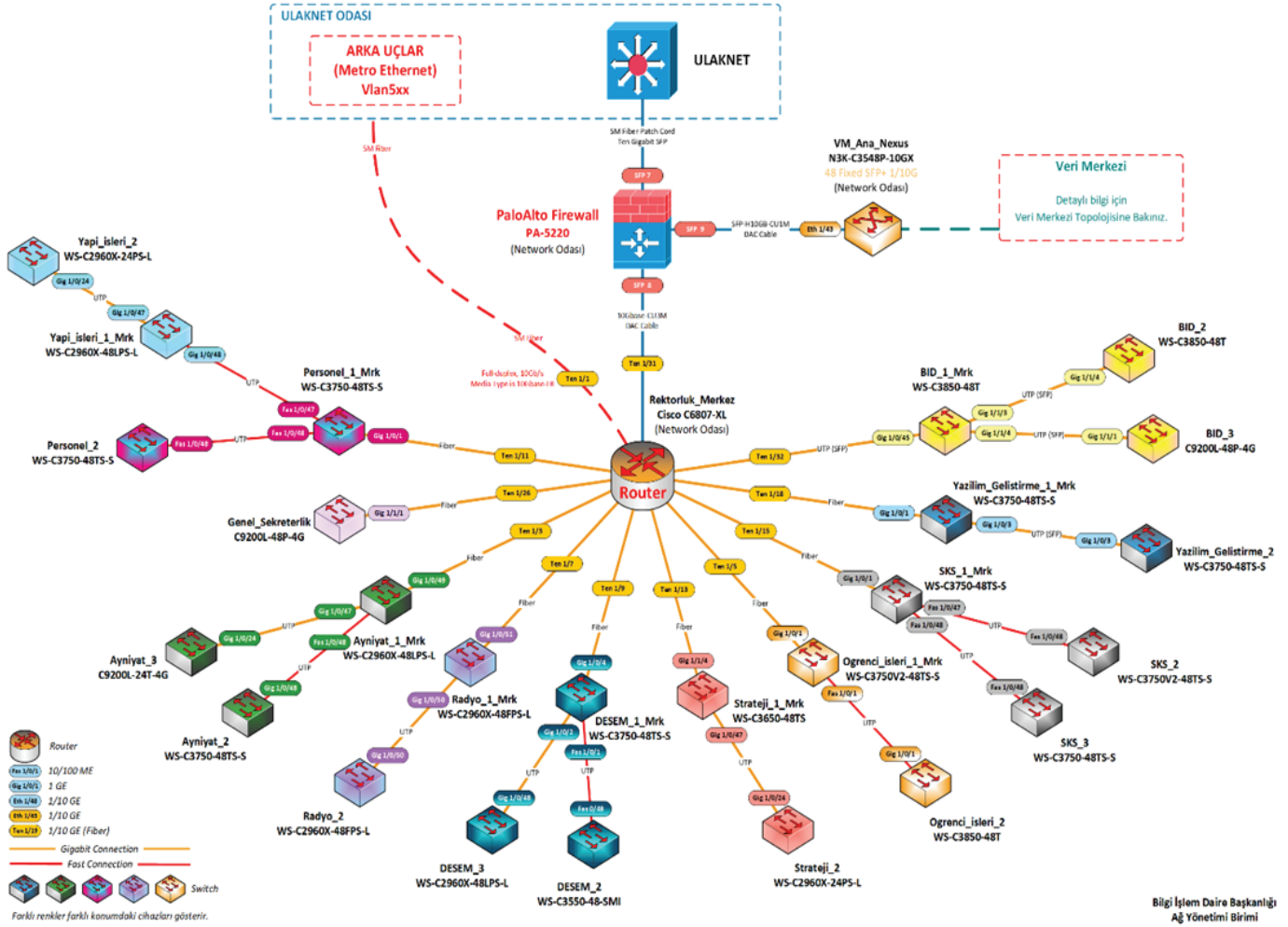
Şekil 5: Birimler Kablolı İnternet Ağı Topolojisi
